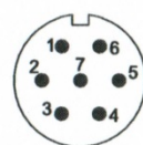
7 POLES
